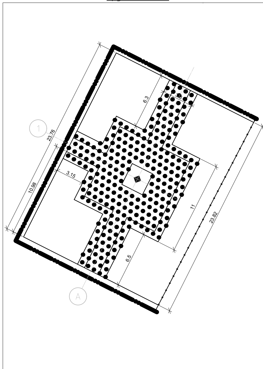
План срезки плодородного грунта М1:200
