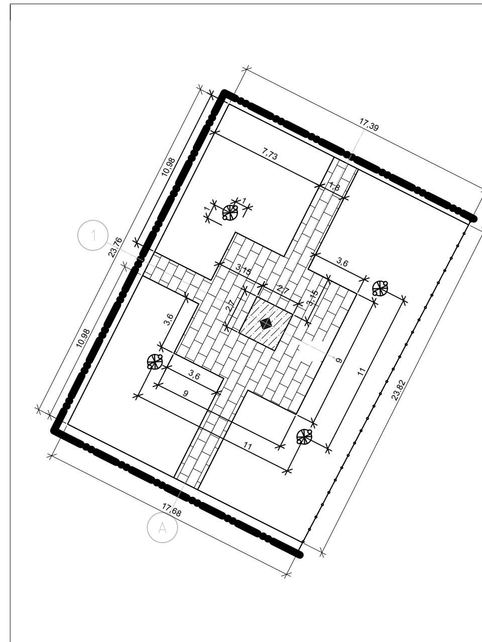
Разбивочный план М1:200
