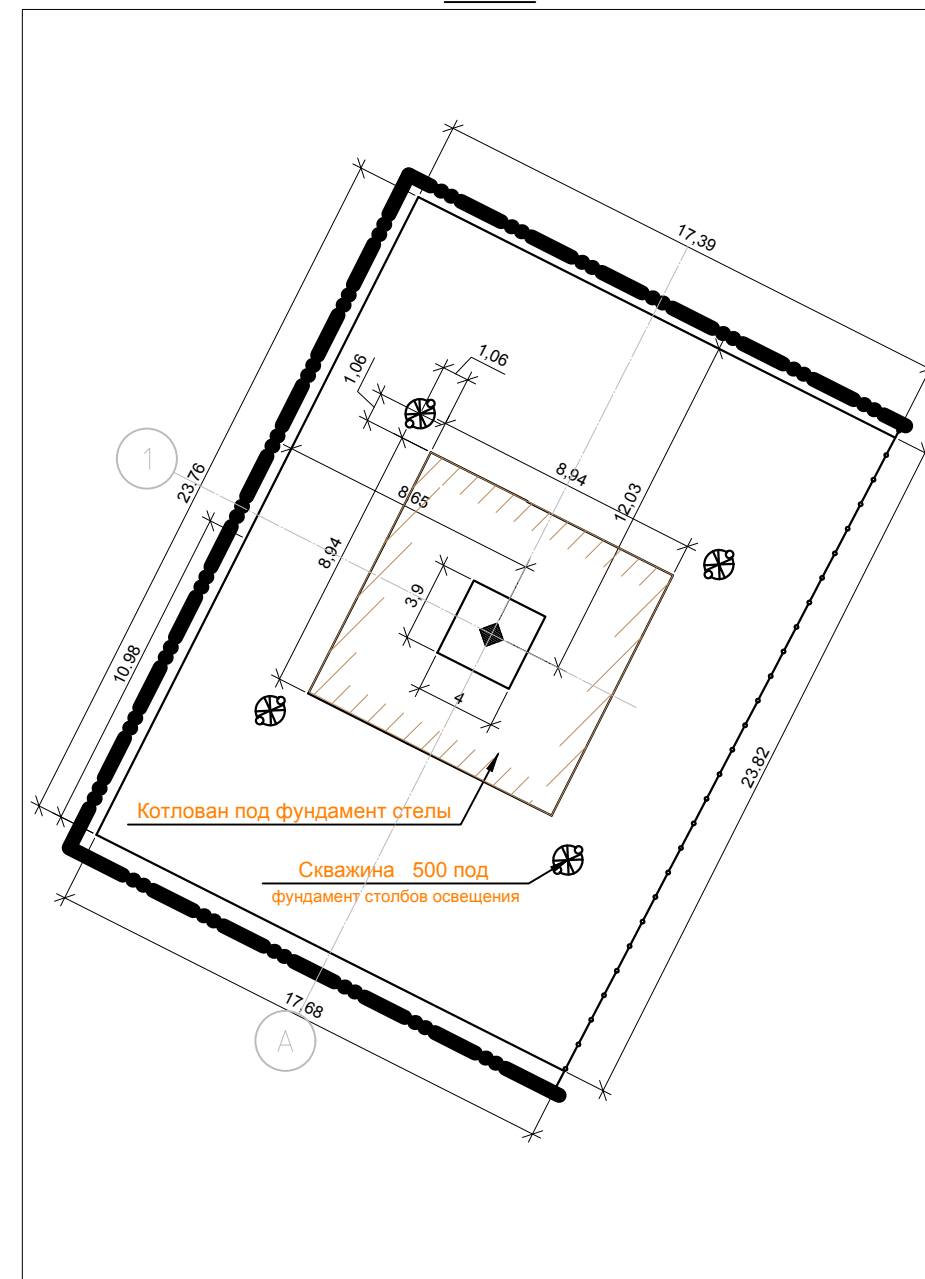
Схема разработки грунта М1:200
