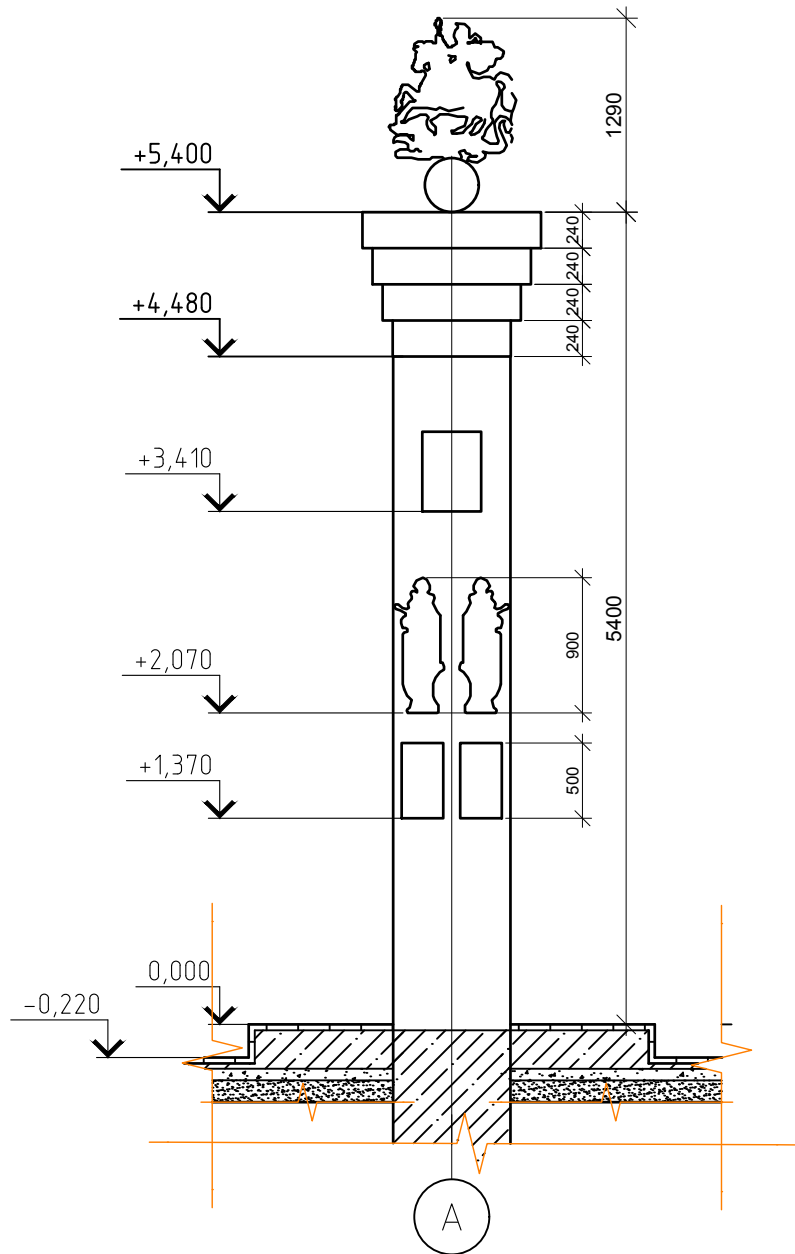
Вид А
