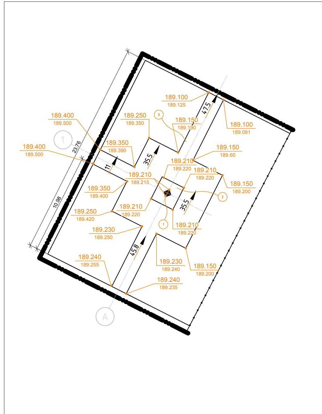
План рельефа М1:200
